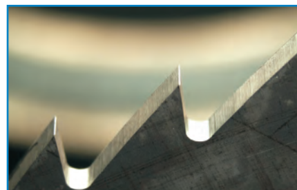
Przykładowy ząb po ostrzeniu
