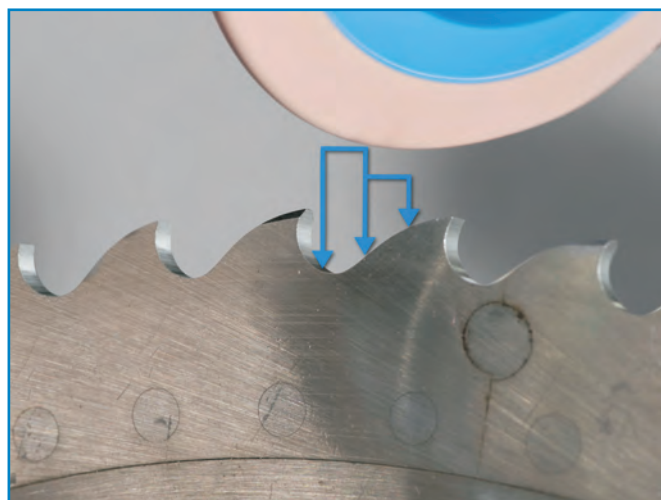
Automatyczne pozycjonowanie ściernicy podczas rozpoznawania średnicy tarczy
