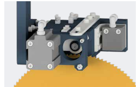
Dispositif d'affûtage brise-copeaux
